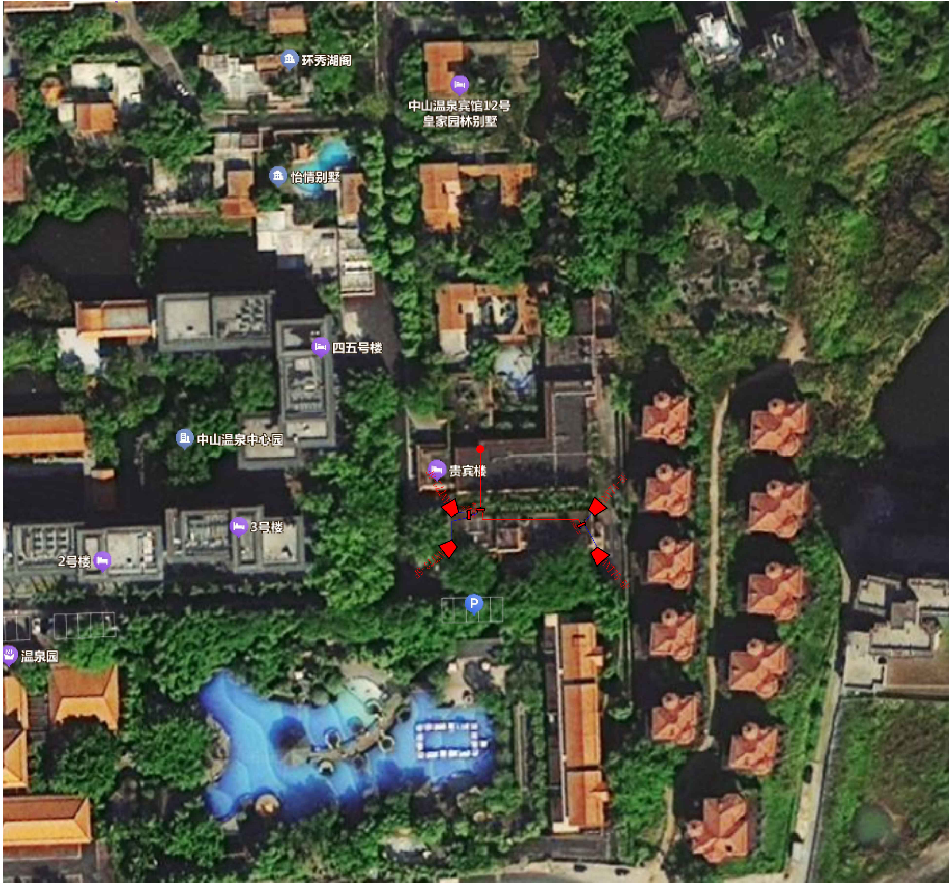
6号楼5F楼顶室外射灯天线安装图
